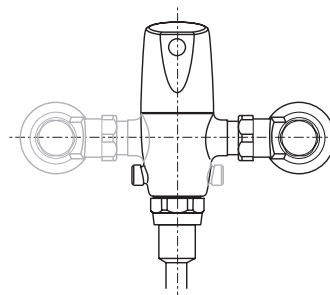
Instalación Derecha o Izquierda
